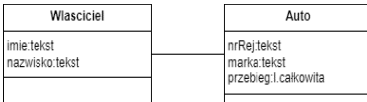
Diagram klas
