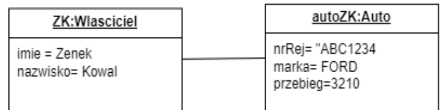
Diagram obiektów
